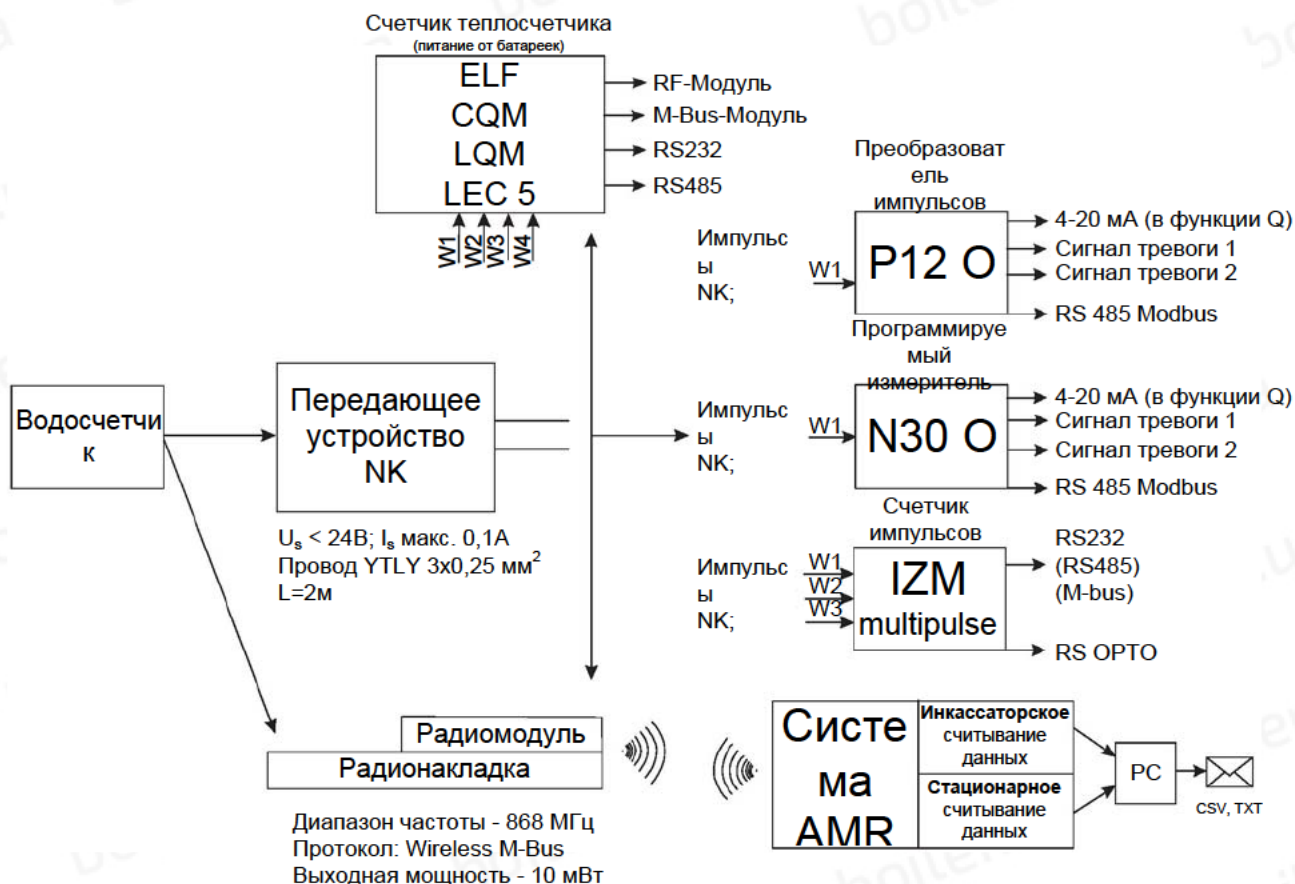
Рис. 5 Схема примерных соединений для осуществления удаленной передачи показаний
