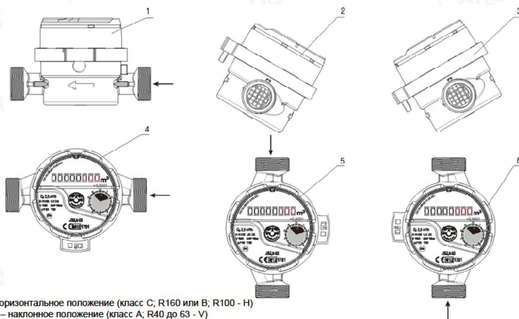
Рис. 1 Примеры допустимых положений установки водосчетчиков производства Apator Powogaz тип JS (DN 15-40).
