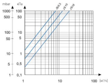
Рис.1 Графіки залежності втрати тиску лічильників від об'ємної витрати
