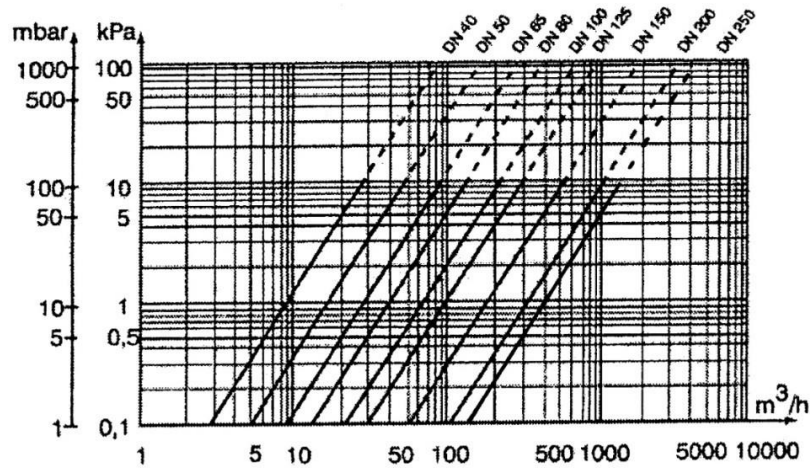
Основні переваги лічильника: Рис. 2 Графіки залежності втрати тиску від витрати води
