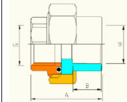
VTр.762 З'єднувач рознімний з переходом на внутрішню різьбу
