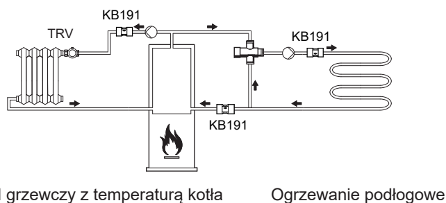
Rys. 1 Standardowy przykład montażu mieszacza termostatycznego
