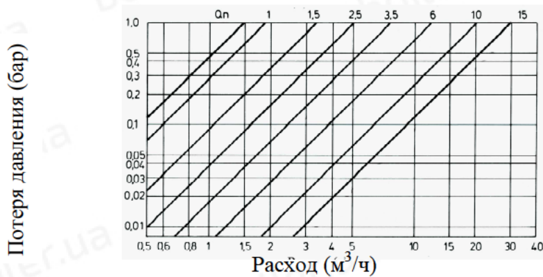
Рисунок 4. Кривая потери давления преобразователя расхода типа RAY FS MT
