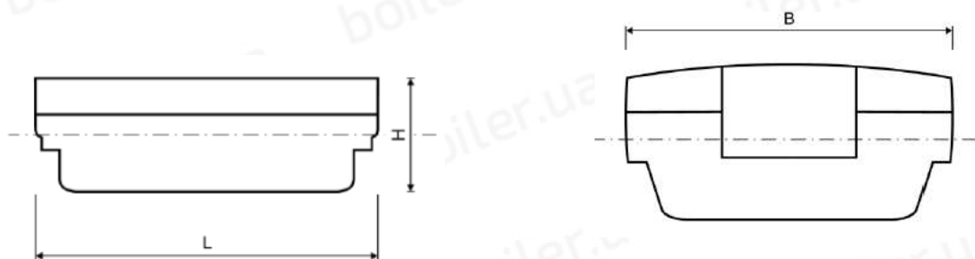
Рисунок 8 - Габаритные размеры тепловычислителя SCYLAR INT 8 ( H=54 мм; B=100 мм; L= 150 мм).
