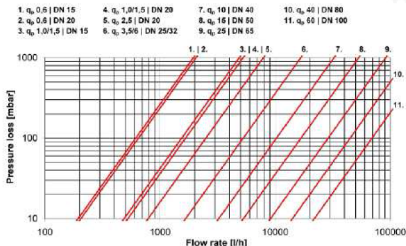
Рисунок 5 - Диаграмма потери давления расходомера SHARKY FS 473
