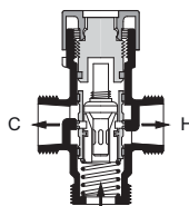
Verdeelventiel
