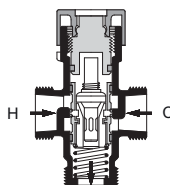
Mengventiel
